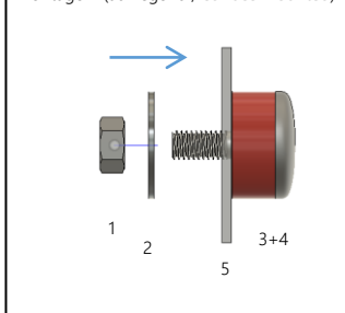
Montage B (aufliegend / surface mounted)
