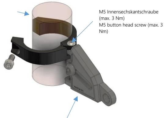
Anbau Beispiel: HIGHSIDER Lampenhalter EXTEND (#220-810)
